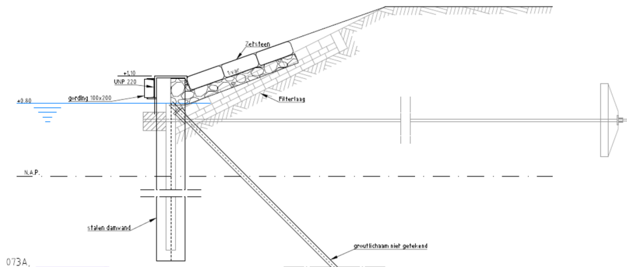
Ontwerp oeverconstructie
