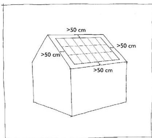
10. Minimaal 50 cm afstand van goot, nok, dakrand, hoekkeper en eventuele dak doorvoeren.
