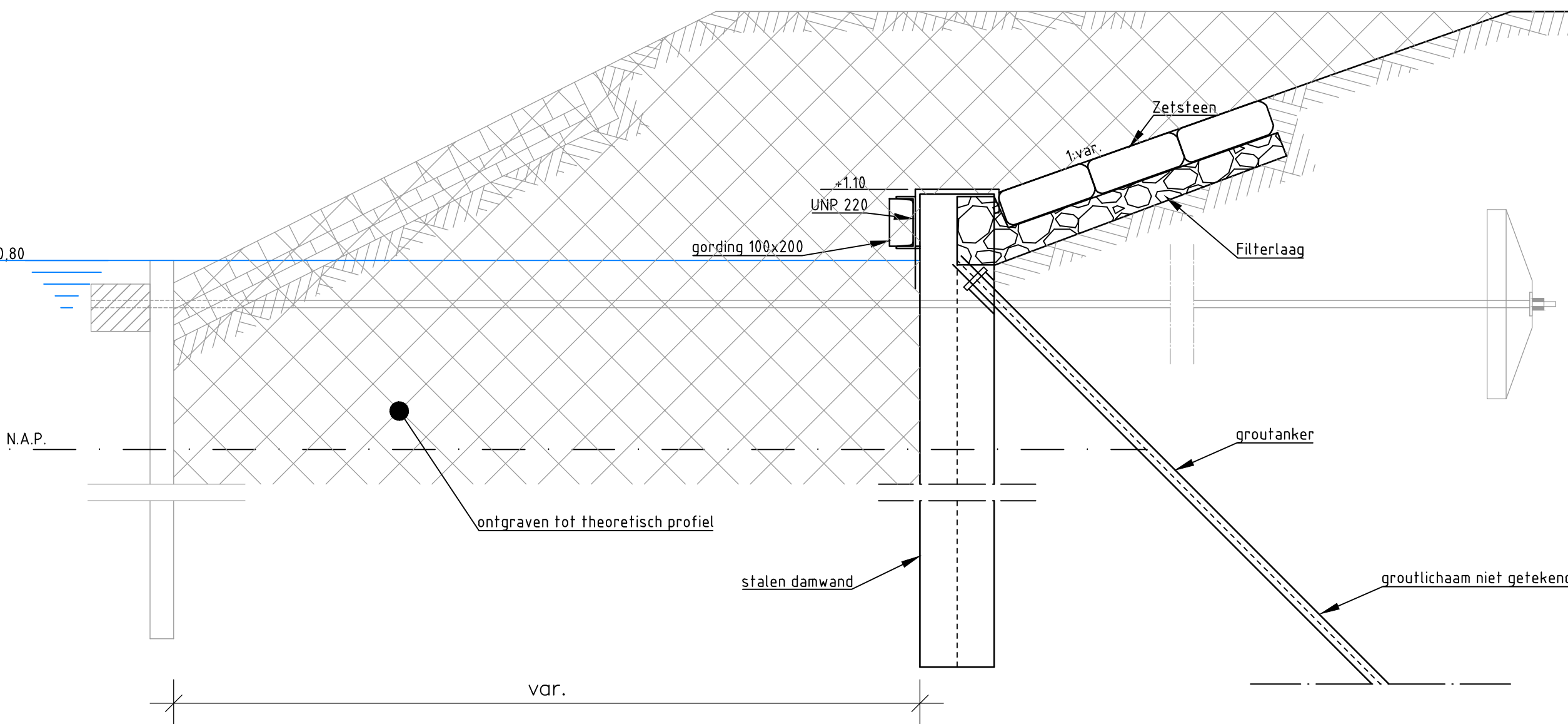
Principeddoorsnede bestaande situatie per oevertype (indicatief) Schaal 1:20
