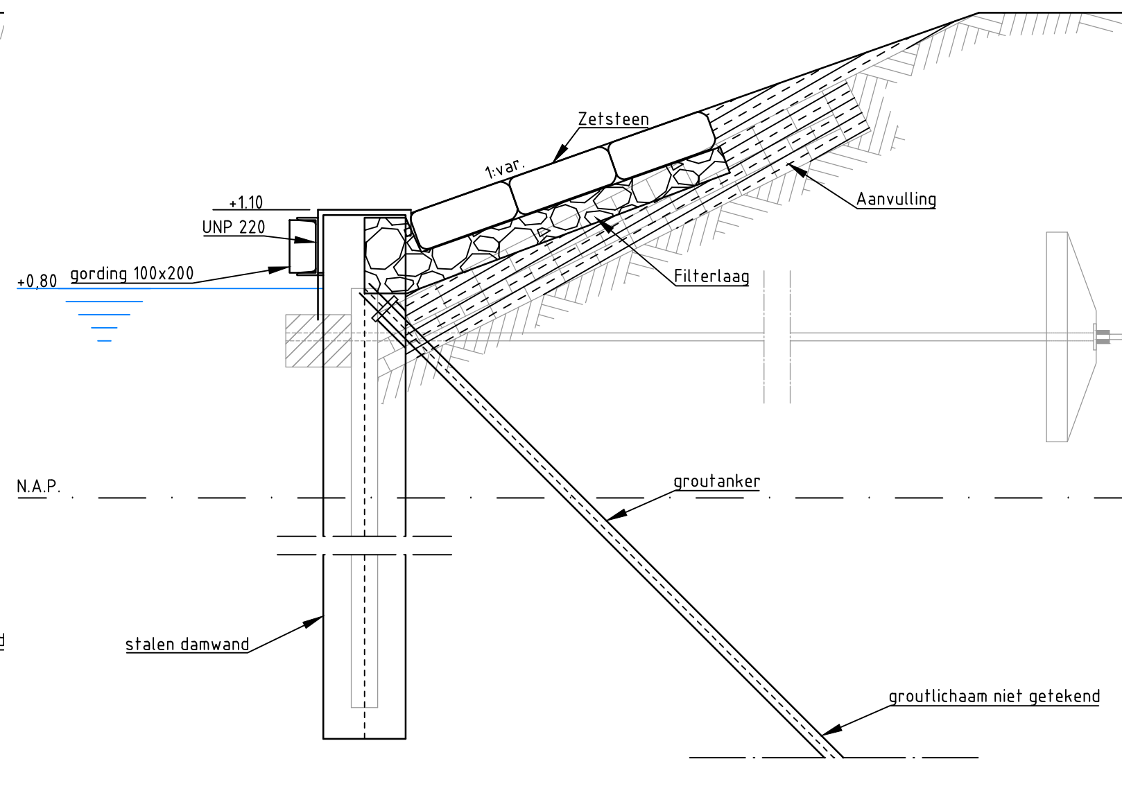
Principeddoorsnede bestaande situatie per oevertype (indicatief) Schaal 1:20
