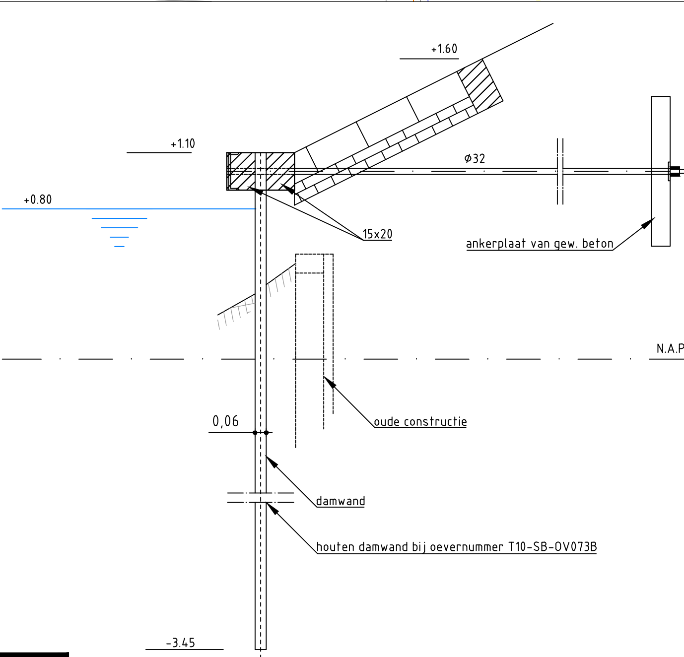
Principeddoorsnede bestaande situatie per oevertype (indicatief) Schaal 1:20
